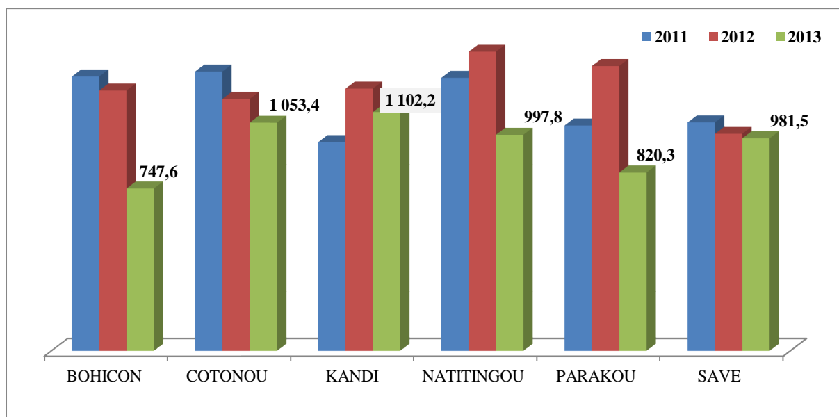
Graphique 11 : Hauteur de pluie (mm) par station en 2011, 2012 et 2013
